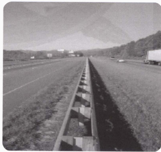
รูปที่ ๖ การติดตั้งราวกันอันตรายแบบรวมเหล็กผูกบนเสาแข็งข้างทางและเกาะกลาง
