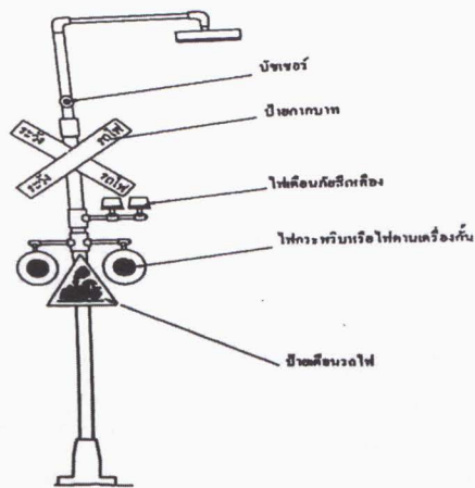
รูปที่ ๖๓ การติดตั้งสัญญาณไฟวบบในกรณีที่ทางตัดผ่านติดตั้งเครื่องกันประเภ้อตโนมัต
