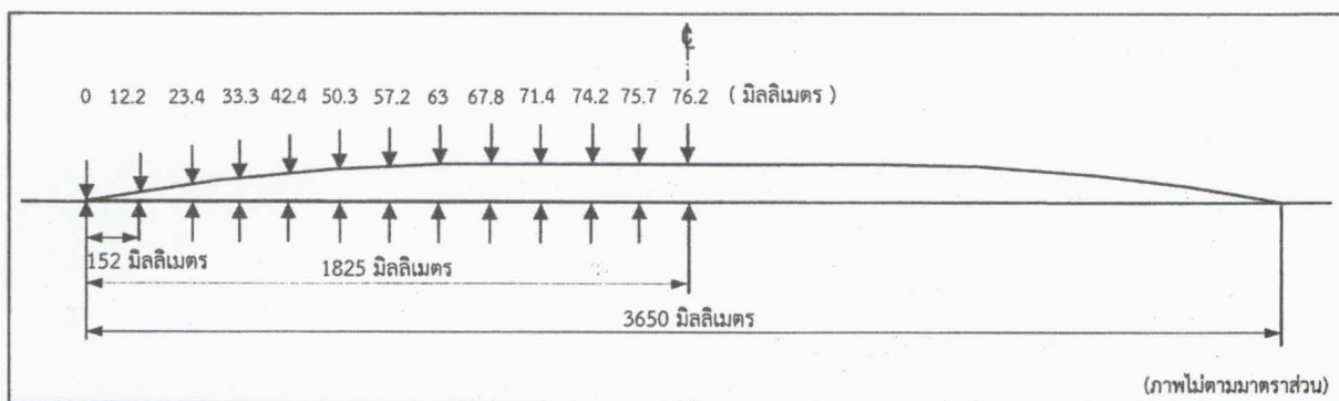
รูปที่ ๖ รูปตัดและขนาดเนินชะลอความเร็วแบบโค้งพาราโบลาแบบ Watts profile hump (ประยุกต์จาก Ewing ๑๙๙๙)
